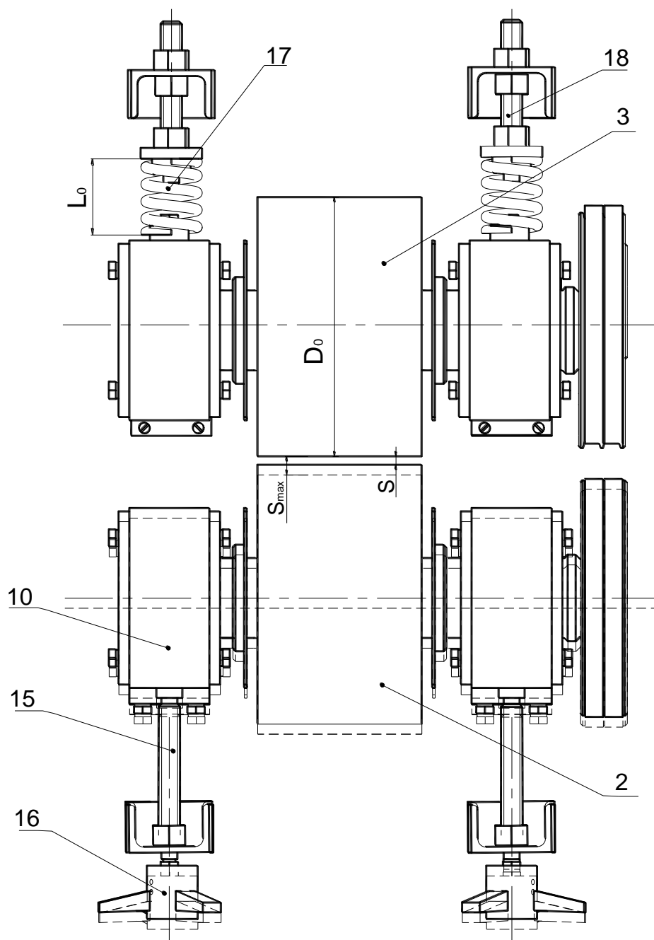
Рис 4. Регулировка зазора между валками.
